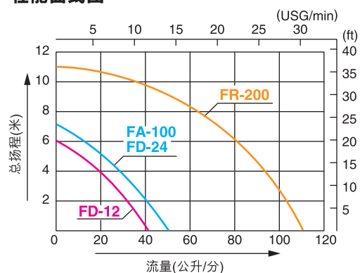
性能曲线图
