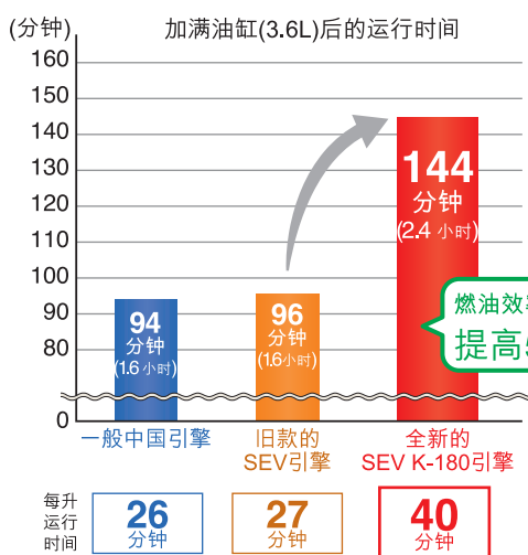
燃油消耗量比较
