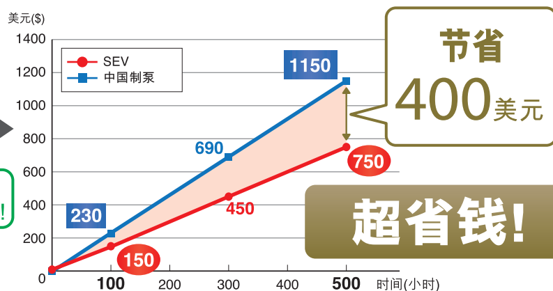
运行成本比较(燃料)
