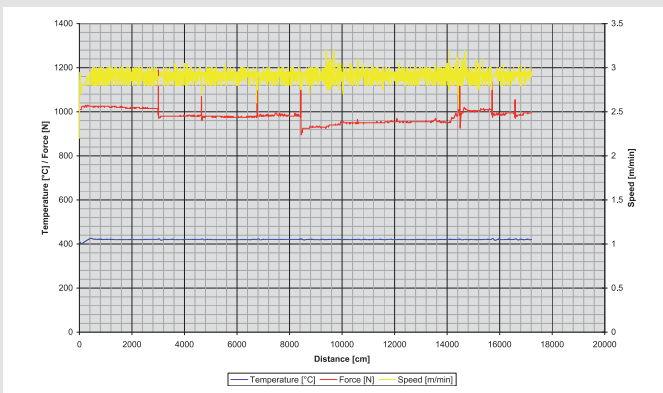
焊缝质量评估图解说明 (焊缝长度: 170 m)。
